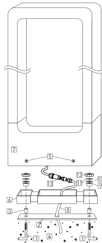
Рис. 1. Установка и подключение светильника.
